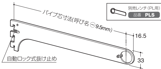
A-79S ハンガーブラケット (外々用)
