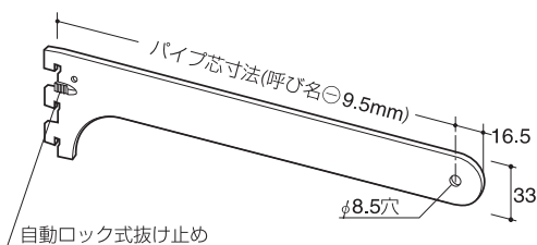
A-78S ハンガーブラケット (内々用)
