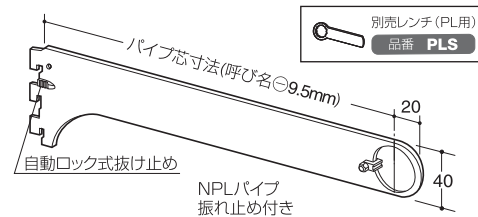
A-80S ハンガーブラケット (外々用)
