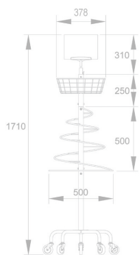
スパイラルスタンド (Aタイプ) + ラウンドバスケット
