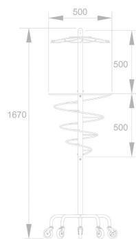
スパイラルスタンド (Bタイプ) + トルネードハンガー
