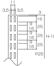
■E支柱断面図 ■E支柱正面図
