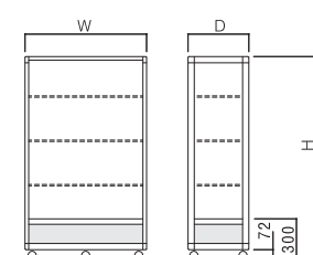
①ハイケースS(腰部ストッカー付) ※棚数: H1800/4段、H2100/5段
