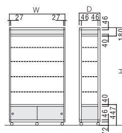
②ハイケースF(腰部FIX) ※棚数: H1800/4段、H2100/5段
