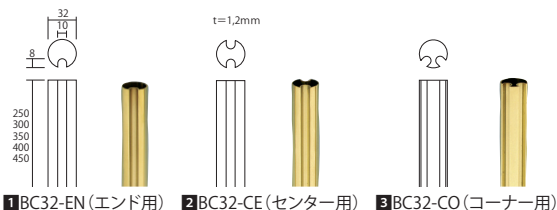
1 BC32-EN (エンド用) 2 BC32-CE (センター用) 3 BC32-CO (コーナー用)
