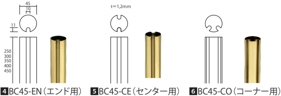
4 BC45-EN (エンド用) 5 BC45-CE (センター用) 6 BC45-CO (コーナー用)
