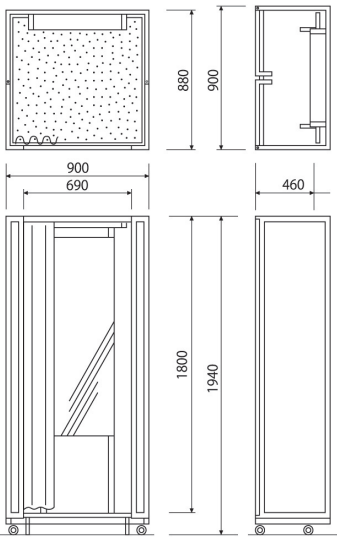
正面図・側面図
