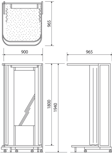
正面図・側面図
