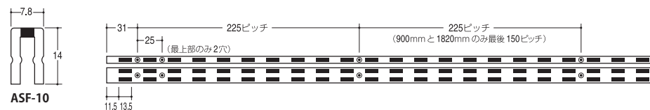
ASF-10 チャンネルサポート
