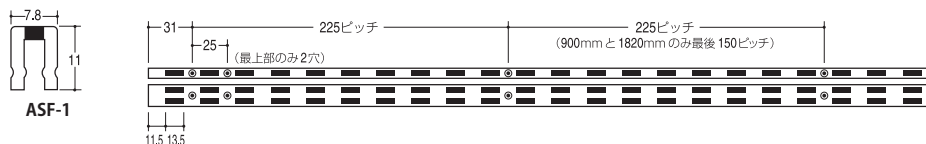
ASF-1 チャンネルサポート
