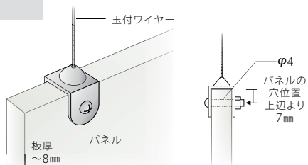
Eタイプセットφ1.0
