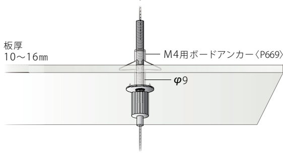
E-9 天井用ロック [φ1.0/1.2]
