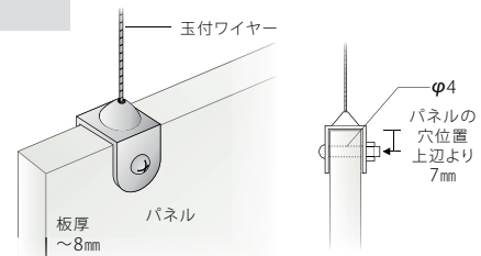
EFタイプセットφ1.0
