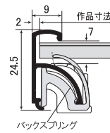
バックスプリング
