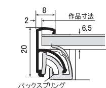
バックスプリング
