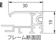
フレーム断面図
