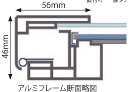
アルミフレーム断面略図
