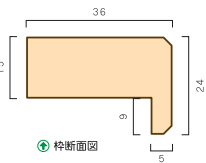
● 枠断面図
