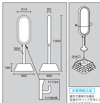
■寸法図 (mm)
