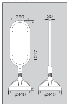
■寸法図 (mm)
