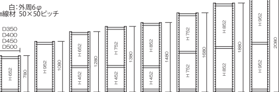
取り付け例
