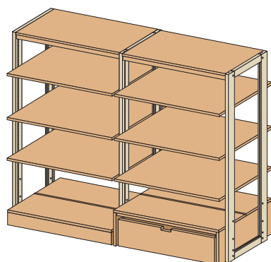
連結例
