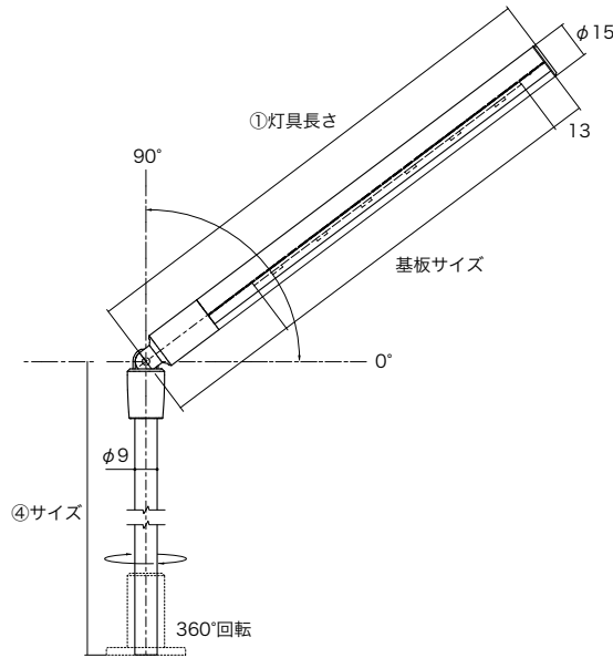
〈灯具断面図〉
