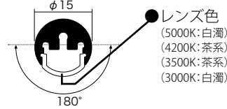
〈灯具断面図〉
