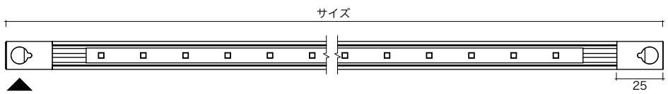
〈灯具平面図〉
