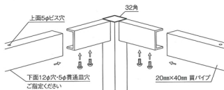
<組立図>
