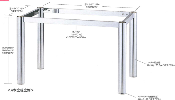
<組立図 コーナー用支柱>
