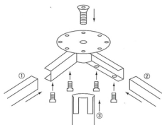
<組立図>
