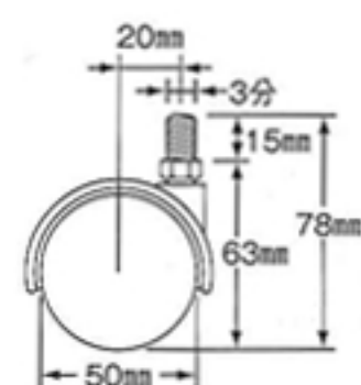
No.319 ナイロン車 許容荷重40kg (ストッパー付) ¥1,100 (ストッパーなし) ¥900 車径50mm
