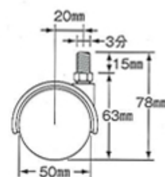
No.311 ナイロン車 許容荷重40kg ¥700 車径50mm
