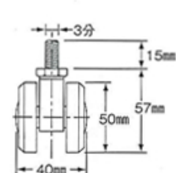
No.322 ナイロン車 許容荷重40kg (ストッパー付) ¥1,100 (ストッパーなし) ¥900 車径50mm
