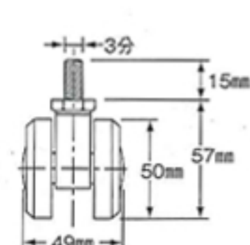
No.321 キャスター ナイロン車 許容荷重60kg ¥900 車径50mm
