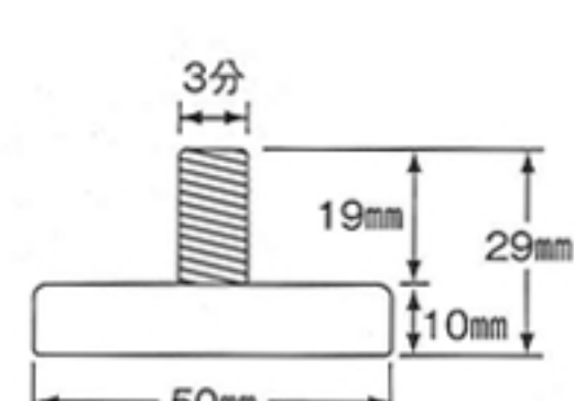
No.315 アジャスター (黒) ¥150 50mmφ×3分ネジ
