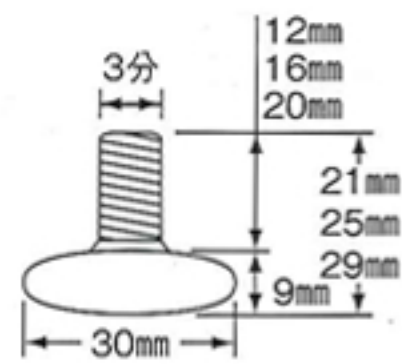
No.316 アジャスター (黒) ¥100 30mmφ×3分ネジ
