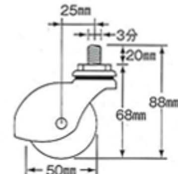
No.313 G型 ゴム車 許容荷重30kg ¥600 車径50mm
