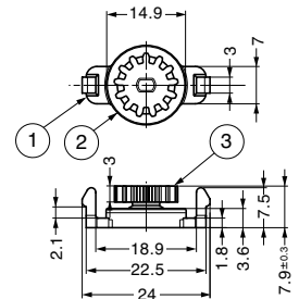
図面は歯数13です
