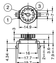
図面は歯数13です
