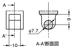
※1 受け側
