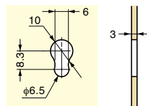
※2 取付側
