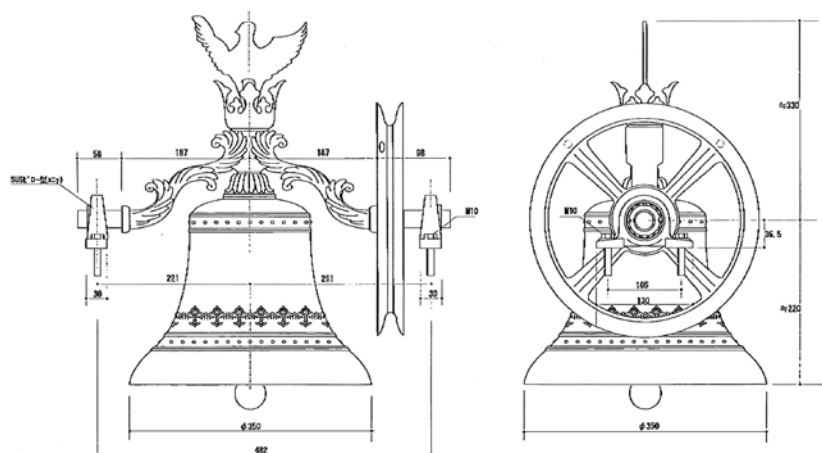
●カリヨン（回転式教会鐘） 寸法図 〈φ 350 39kg〉の例
