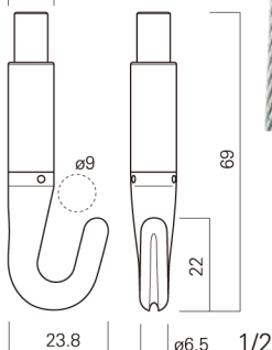
Nハンガー N hanger
