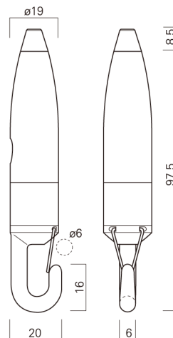
P2ハンガー P2 hanger
