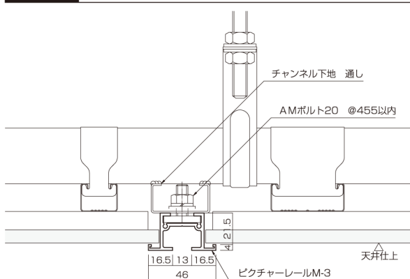
M - 3 天井中間 取付例 Ceiling installation
