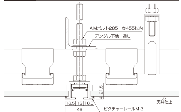
M - 3 天井中間部埋込み 取付例 Ceiling installation
