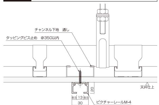
M - 4 天井中間 取付例 Ceiling installation
