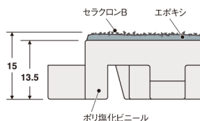
側面形状
