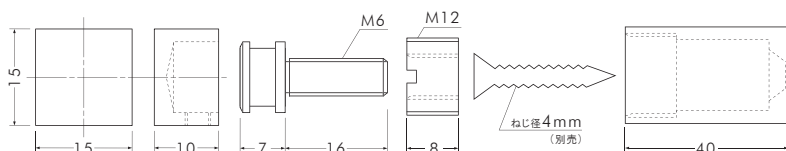
SCP-AA382 / □15-40
