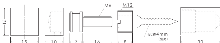
SCP-AA381 / □15-30
