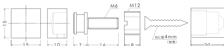
SCP-AA380 / □15-20
