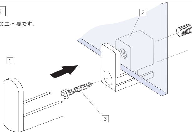
取付図
