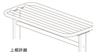
上棚詳細
