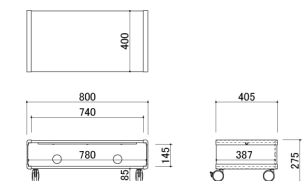
TVR-8040
