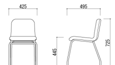
MU-4M-C □□
