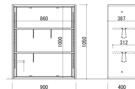
TJ書庫 ※図中W・D・Hは有効内寸法
