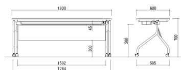
AHM-1860 AHM-JM1860
